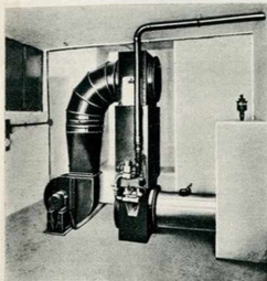
Générateur type G.P.50 de 50.000 calories/heure (Groupe échangeur de température avec son moto-ventilateur).
