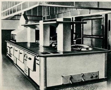
Installation de cuisine au gaz, avec 4 marmites encastrées, friturier, 2 feux vifs, 2 grandes plaques de coup de feu, 4 fours, grillade double et étuve, réalisée au Pensionnat de l'Immaculée Conception, à Laval (350 repas).
